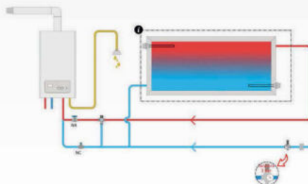
Collegamento idraulico con generatore di calore predisposto per integrazione solare
