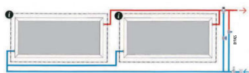
Collegamento di più collettori in parallelo.
