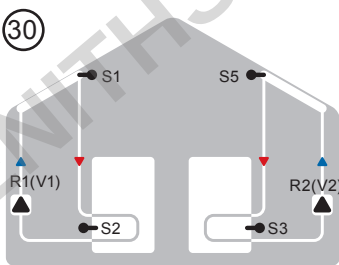
Doppio solare
