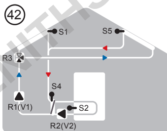
Solare est-ovest, scambiatore e 2 pompe
