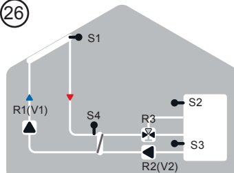
Solare con scambiatore 2 zone
