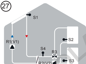
Solare con scambiatore 2 accumuli
