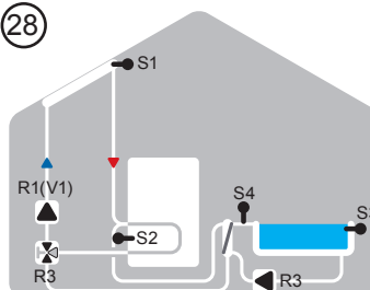
Solare piscina, accumulo, scambiatore
