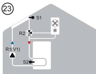
Solare + raffreddamento 1
