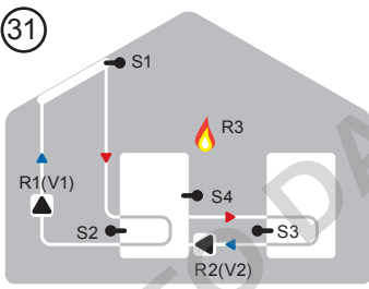
Solare con termostato e trasferimento
