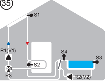
Solare con piscina, accumulo, scambiatore
