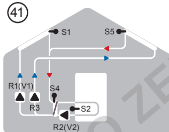
Solare est-ovest, scambiatore e 3 pompe
