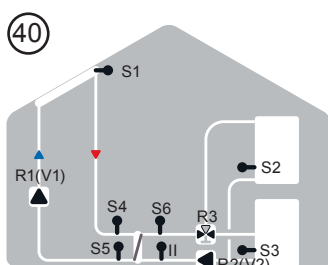
Solare con scambiatore e 2 accumuli
