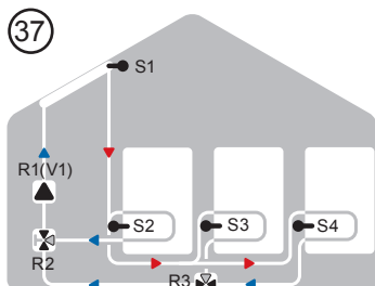
Solare 3 accumuli e 3 valvole
