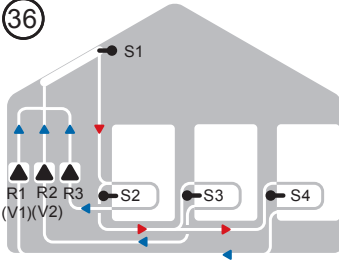
Solare con 3 accumuli e 3 pompe
