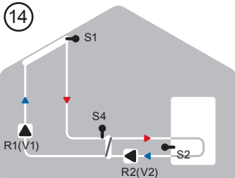
Solare + scamb.
