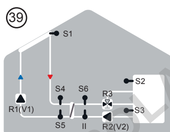
Solare con scambiatore e 2 zone
