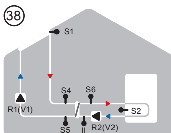
Solare con scambiatore
