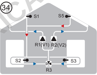
Solare est-ovest, 2 accumuli, 2 pompe
