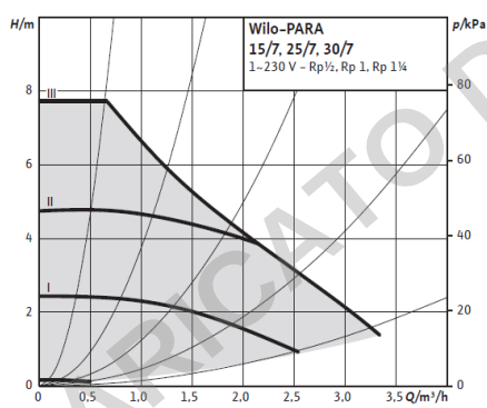
Diagramma giri costanti
