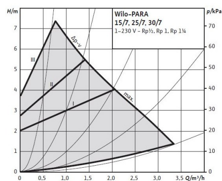
Diagramma pressione variabile
