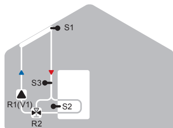
Solare + bypass
