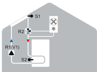
Solare + raffreddamento 1
