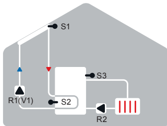
Solare + raffreddamento 3
