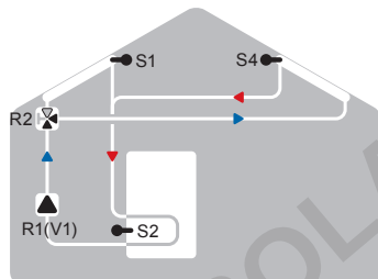
Solare + 2 collettori
