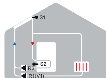
Solare + raffreddamento 2
