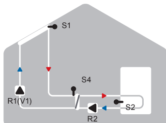
Solare + scamb.
