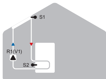
Solare
