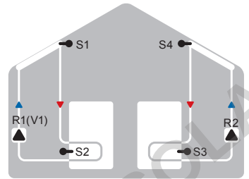
Doppio solare
