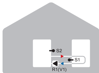
Trasferimento
