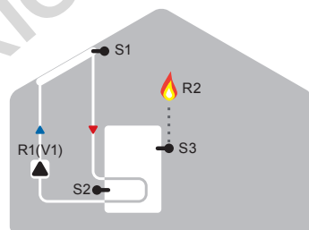
Solare + termostato
